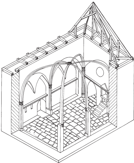
Marburg, Markt 24. Isometrische Rekonstruktion der Synagoge in Phase III mit Blick nach Osten (Freies Institut für Bauforschung, IBD 2000)/ Marburg, Markt 24, isometric reconstruction of the synagogue in phase III toward east (IBD 2000).
